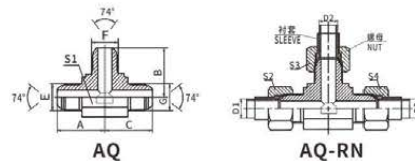
公制外螺纹74° 外锥三通 METRIC MALE 74° CONE TEE
