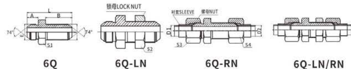
公制外螺纹74°外锥过板接头 METRIC MALE 74° CONE BULKHEAD
